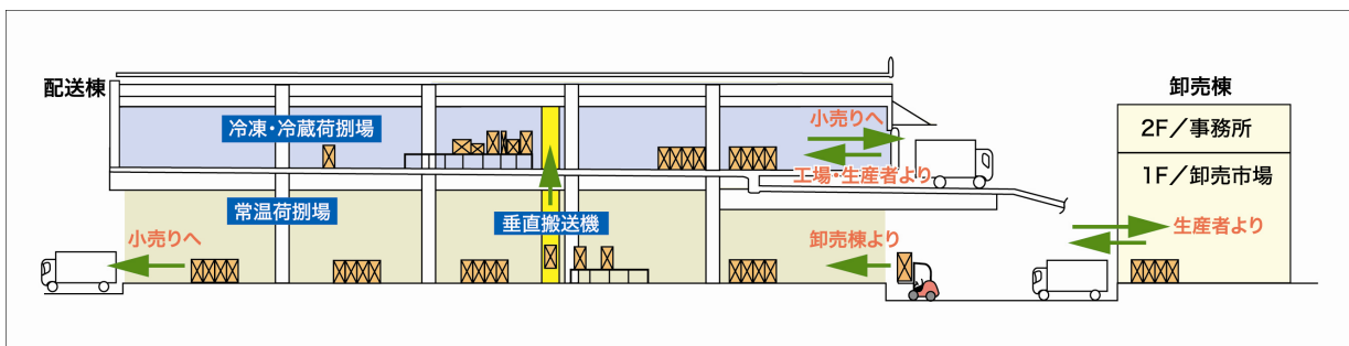
断面レイアウト
