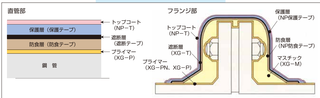
【NP防食工法の構造】
